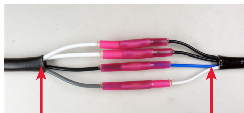
Stecker der OE Lambdasonde Nr.3
